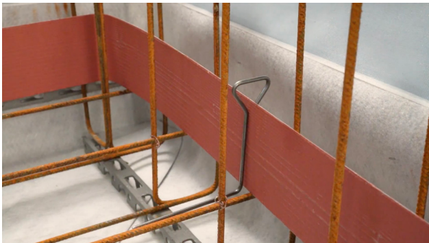
Fixieren mit Bindedraht
